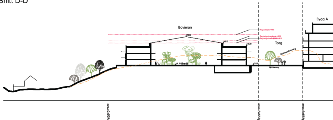
Fig.30. Felt BB1 – Landskapssnitt som viser Bovieran og byggets plassering i terrenget, og forskjellen mellom eksisterende og nytt terreng. Eksisterende terreng har store variasjoner innenfor delfeltet
